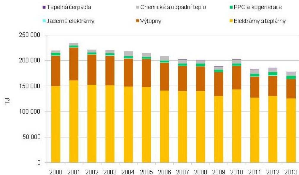
Graf 3 → Čistá výroba tepla podle zdroje v ČR [TJ], 2000–2013
