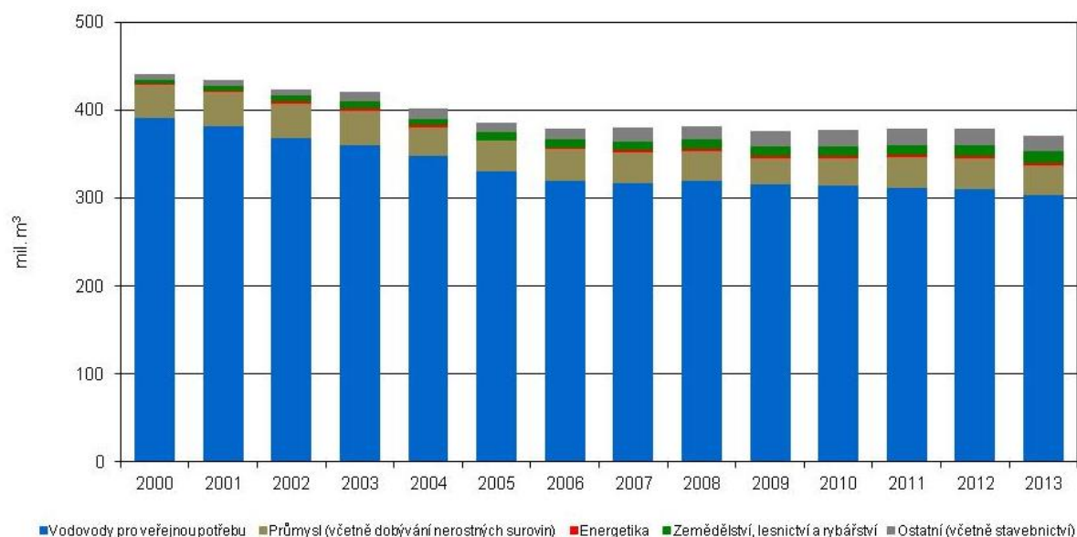
Graf 2 → Odběry podzemní vody jednotlivými sektory v ČR [mil. m 3 ], 2000–2013
