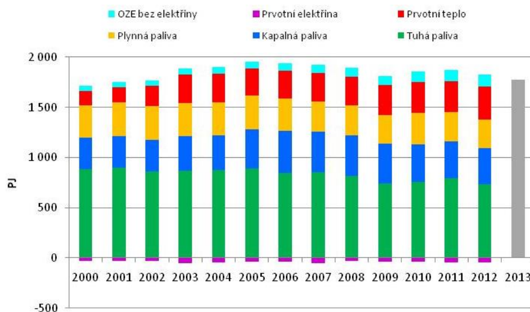
Graf 2 → Vývoj spotřeby primárních energetických zdrojů v ČR [PJ], 2000–2013
