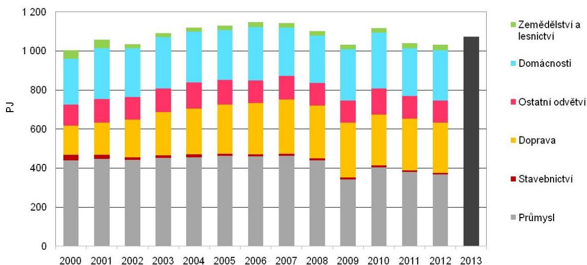
Graf 2 → Vývoj konečné spotřeby energie dle odvětví v ČR [PJ], 2000–2013
