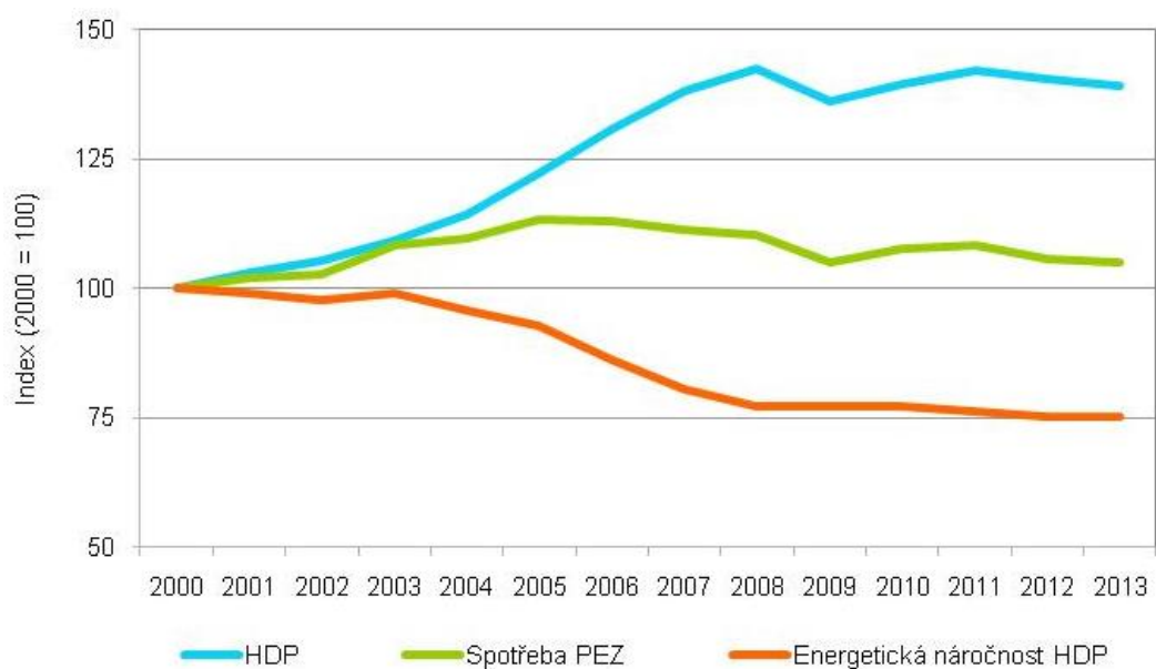
Graf 1 → Energetická náročnost HDP v ČR [index, 2000 = 100], 2000–2013
